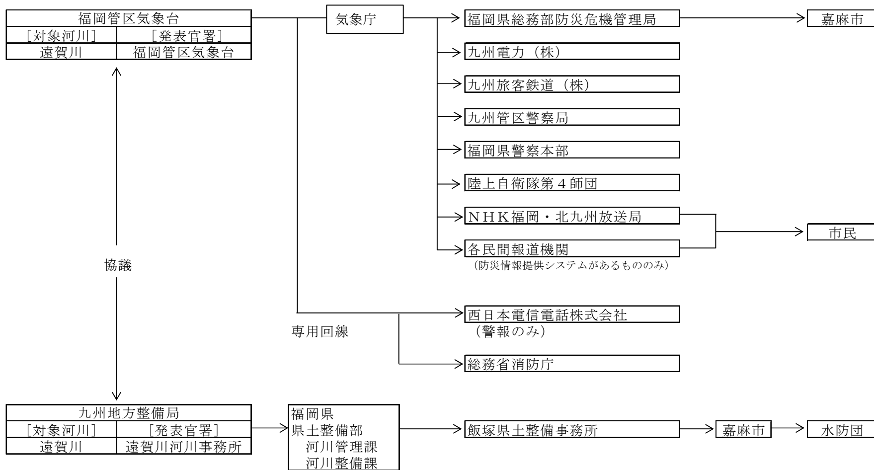
(2) 伝達系統図
