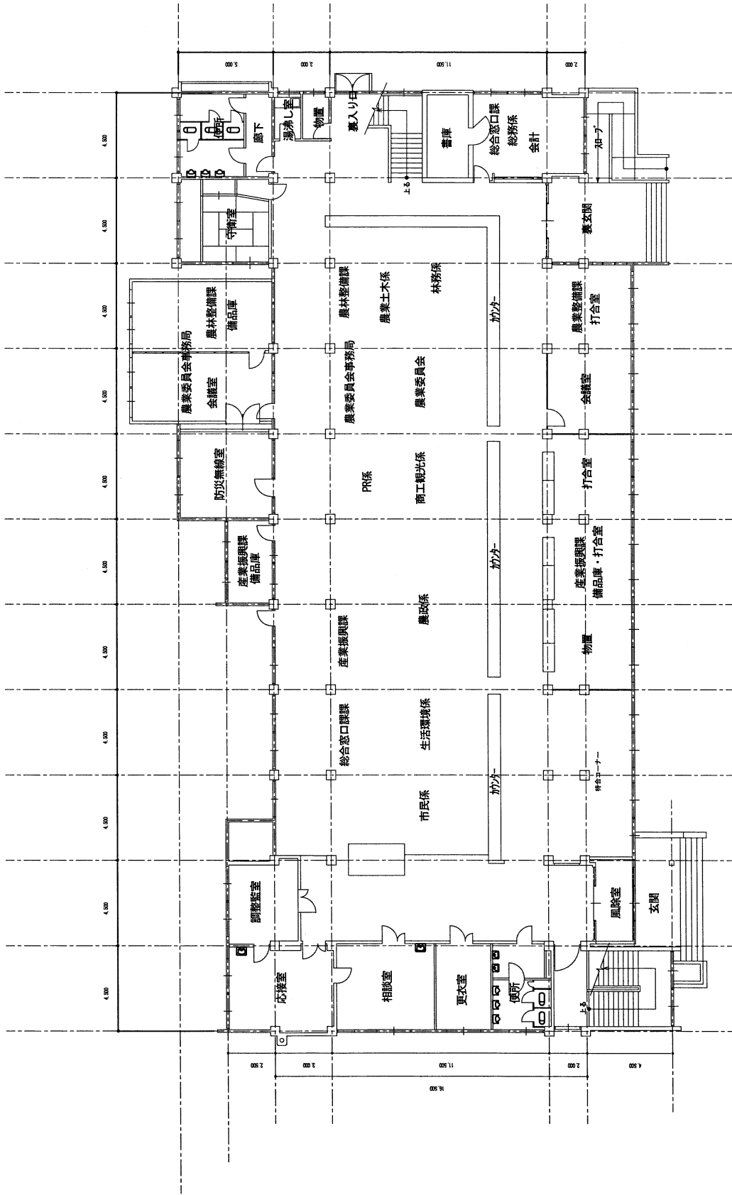
嘉穂庁舎 1階平面図
