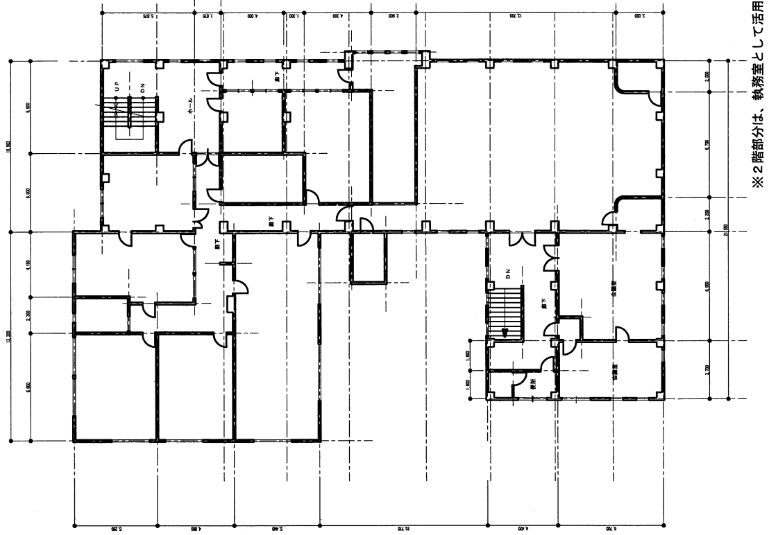
2階平面図
