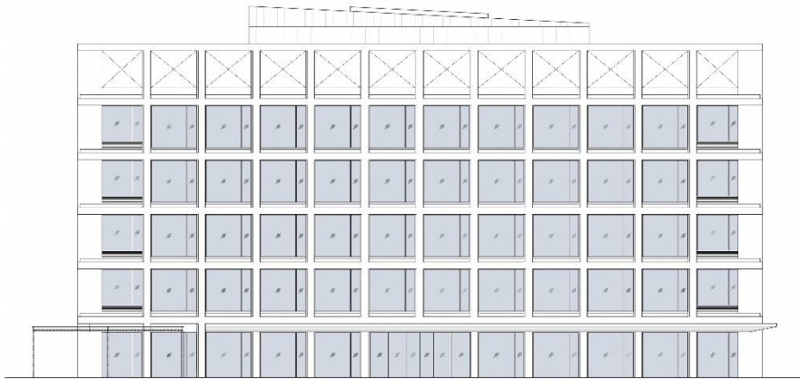
△新庁舎立面図(西)
