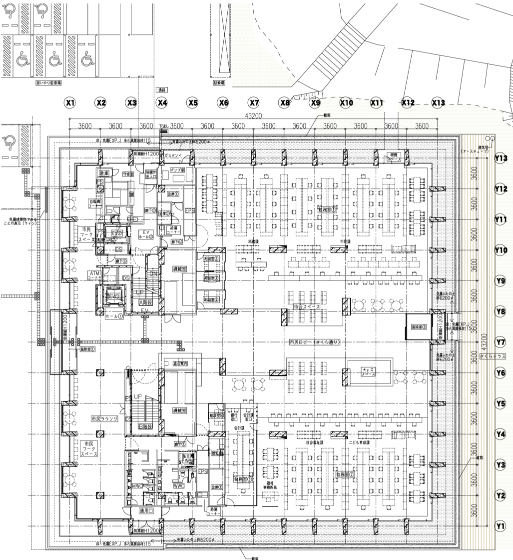
1階平面図
