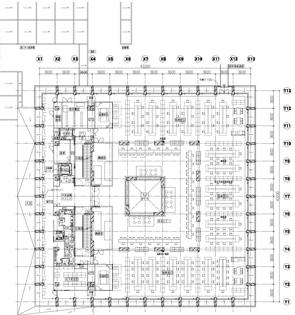
2階平面図
