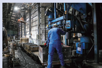
鋳造に必要な砂型の製造工程。
