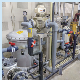
▲出荷前の状態の水処理用FRP製ろ過タンクです。
