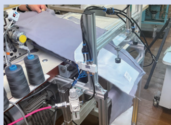
▲自社開発の自動送り機
