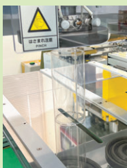
▲円筒ケース成型機 筒状の上下(端部分)を丸く加工します。
